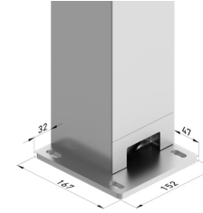
Soporte suelo módulo simple Single module floor support
