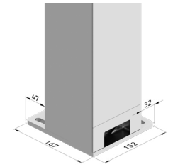
Soporte suelo módulo simple a muro Single module floor-to-wall support
