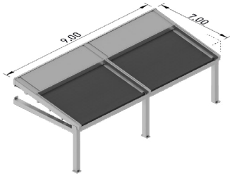
Módulo Doble Double Module
